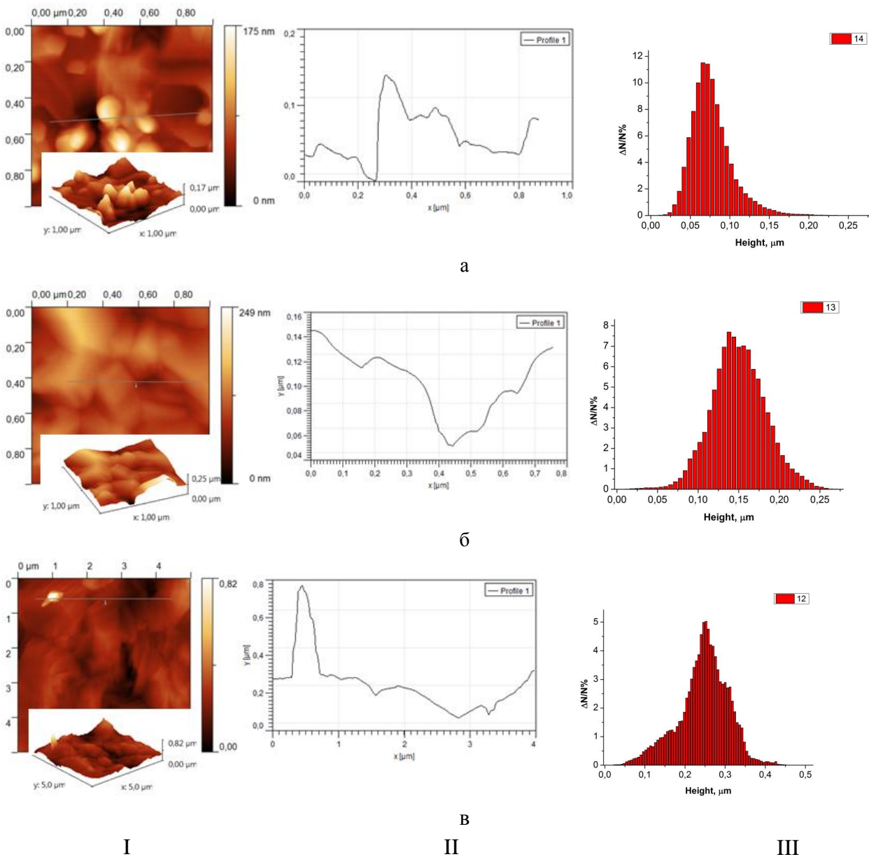
Рис. 3. АСМ – зображення (I), профілограми (II) і гістограми висот (III) наноструктур CdTe на підкладках скла при різному часі осадження t_d , хв: 0,5 (а), 1 (б), 5 (в); T_B=500 °C, T_C=550 °C, T_H=250 °C.
