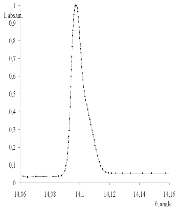
Рис. 2. Крива «гойдання», отримана від поверхні окисненого кремнію КЭФ-4.5 (100), виміряна за допомогою двохкристалльного дифрактометра ДРОН -2 (товщина оксиду кремнію 1,5 мікрон).
