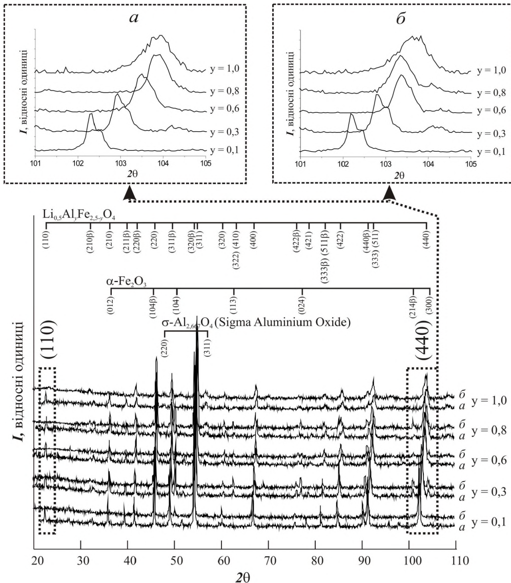
Рис. 1. Дифрактограми серій зразків. На вставках – рефлекс (440) для зразків: a – серія №1; б – серія №2.
