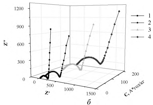
Рис. 12. Діаграми Найквіста від електрохімічної комірки при y = 0,8 для зразків: a – серія №1; б – серія №2.
