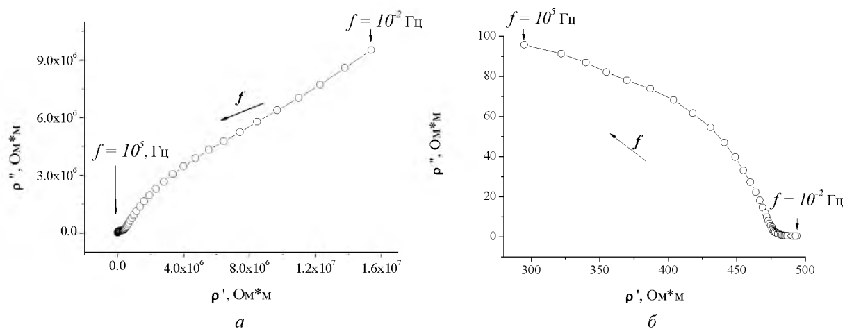
Рис. 5. Діаграми Найквіста для питомих значень комплексного імпедансу досліджуваних зразків при y = 0,8 для зразків: а – серія №1; б – серія №2.
