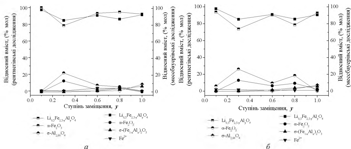
Рис. 4. Фазовий склад синтезованих зразків, визначений X-проміневим та мессбауєрівським методами для зразків: а – серія №1; б – серія №2.
