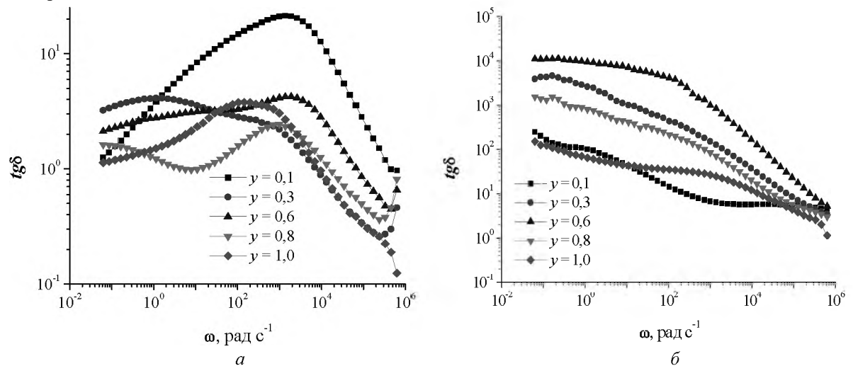
Рис. 9. Частотні залежності діелектричних втрат tg\delta системи для зразків: а – серія №1 ; б – серія №2 .
