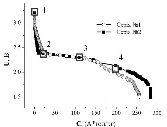
Рис. 11. Експериментальні розрядні криві електрохімічних комірок з катодами на основі синтезованих систем при y = 0,8 .
