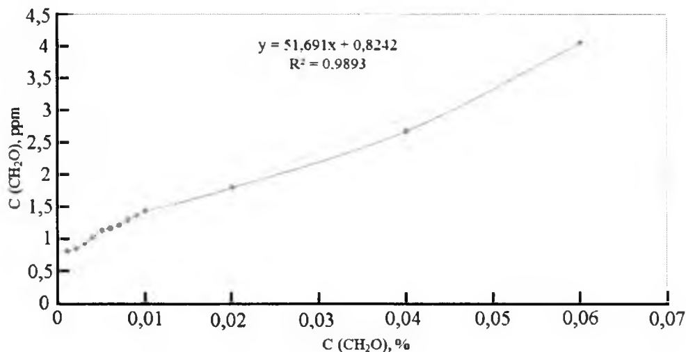
Рис. 2. Калібрувальний графік залежності визначеної приладом масової частки ррп метаналу у насиченому ним повітрі від масової частки метаналу у водному розчині.
