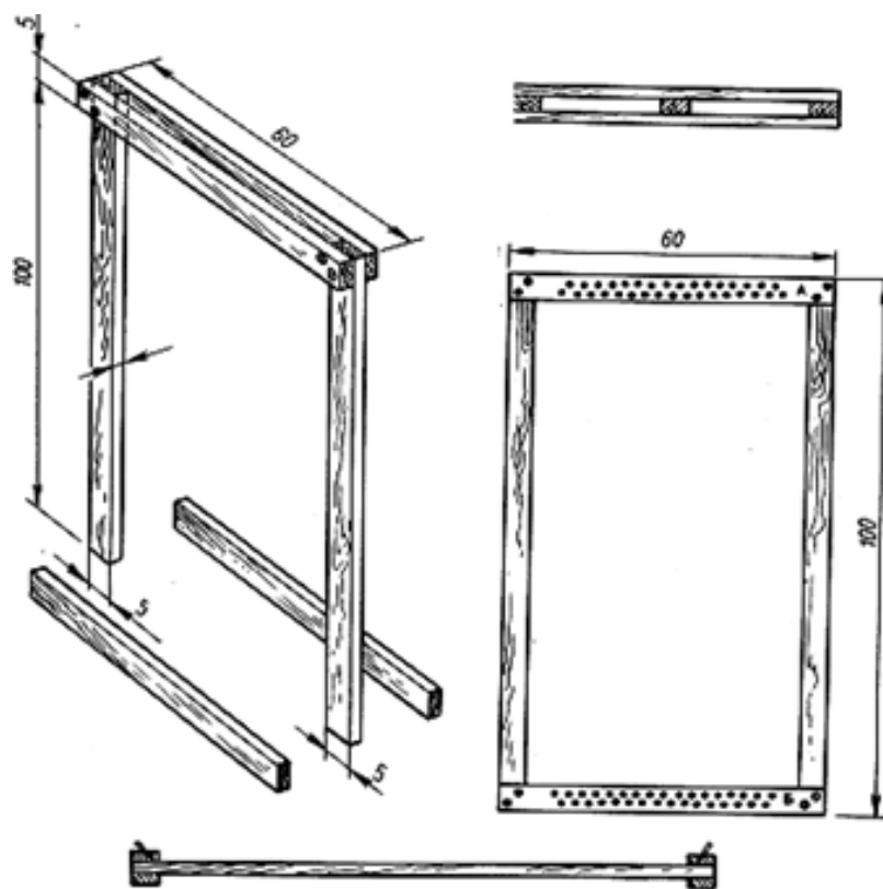
Ткацька рама із набитими цвяшкамі у два ряди
