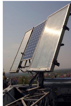
Рис. 3. Система «Сонячний колектор – фотовольтаїчна панель».
