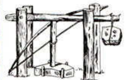
Варштат для свідравання каменю
