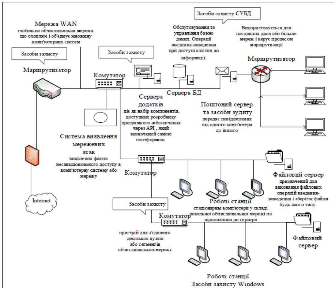
Рис. 2. Структурна схема підсистеми захисту інформації в СЕП
